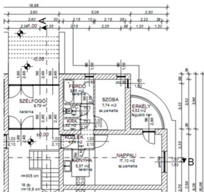
Egy földszinti lakás alaprajza.
